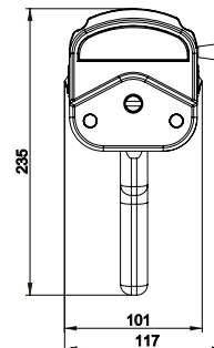
正视图
